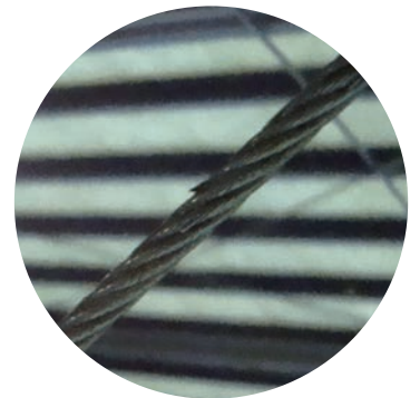
吊り上げワイヤー極度摩耗
