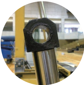
クレビス用ねじ棒変形
